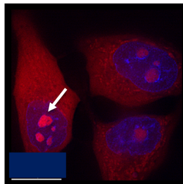
RNA（核小体） イメージング蛍光色素
