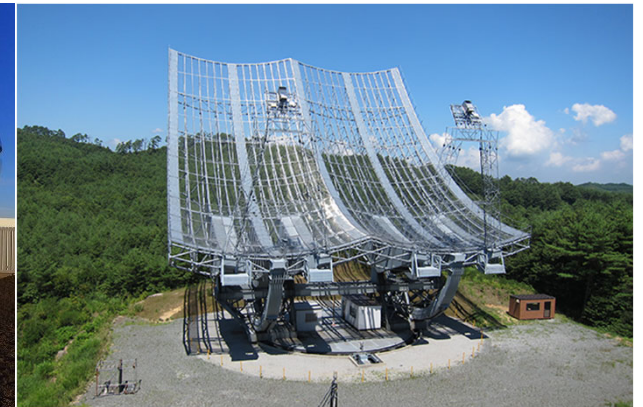
宇宙地球物理 ：天体観測所 (ハワイマウイ島) 大型電波望遠鏡 (福島県飯舘村)
